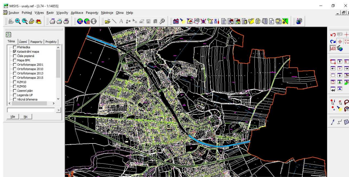
Obr. 3: Prostředí MISYS
