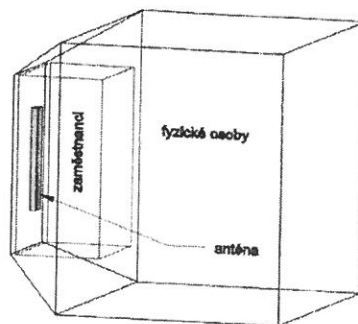
Axonometrie zóny pro panelové antény
