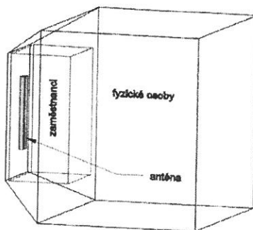
Axonometrie zóny pro panelové antény
